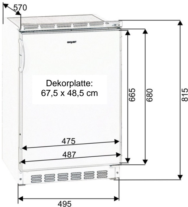
Unterbau-skizze
